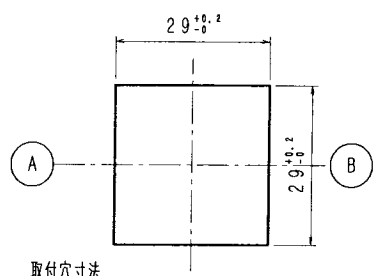
取付穴寸法
